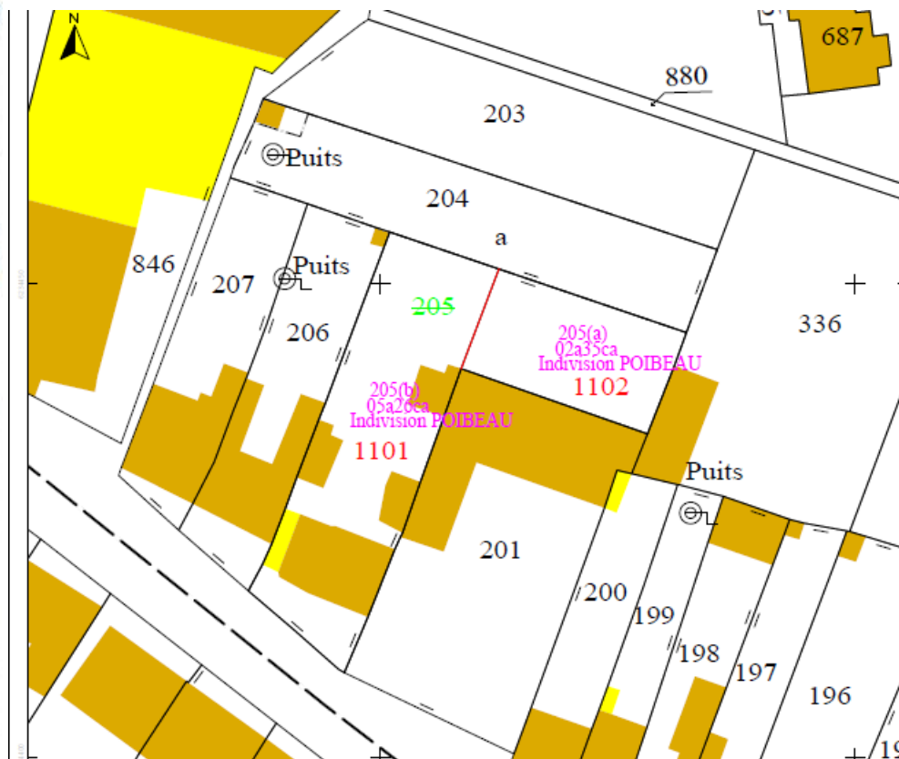
PLAN DE BORNAGE
